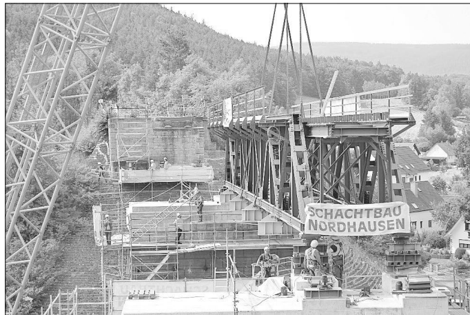
Im Juli 2013 wird das erste überholte Segment wieder auf den Pfeilern montiert.
