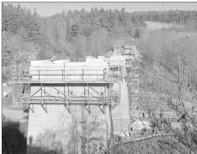
Im November 2012 war Ruhe an der Brücke. Gut zu erkennen sind die erneuerten Brückenköpfe.
